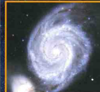
Galaxie du Tourbillon
