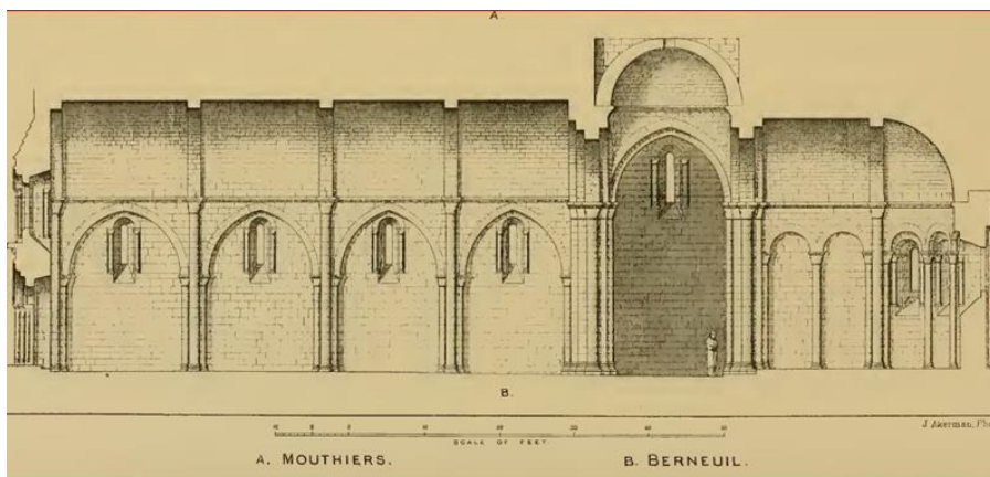
L'église Notre Dame de Berneuil en 1875, coupe : Edmund Sharpe
