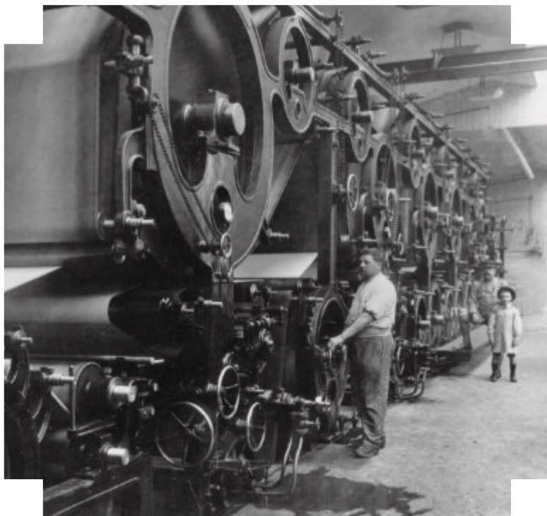
Machine III fonctionnant à Cran en 1915. Collection Aussedat ©Fonds de la photothèque des Musées d'Anncy
