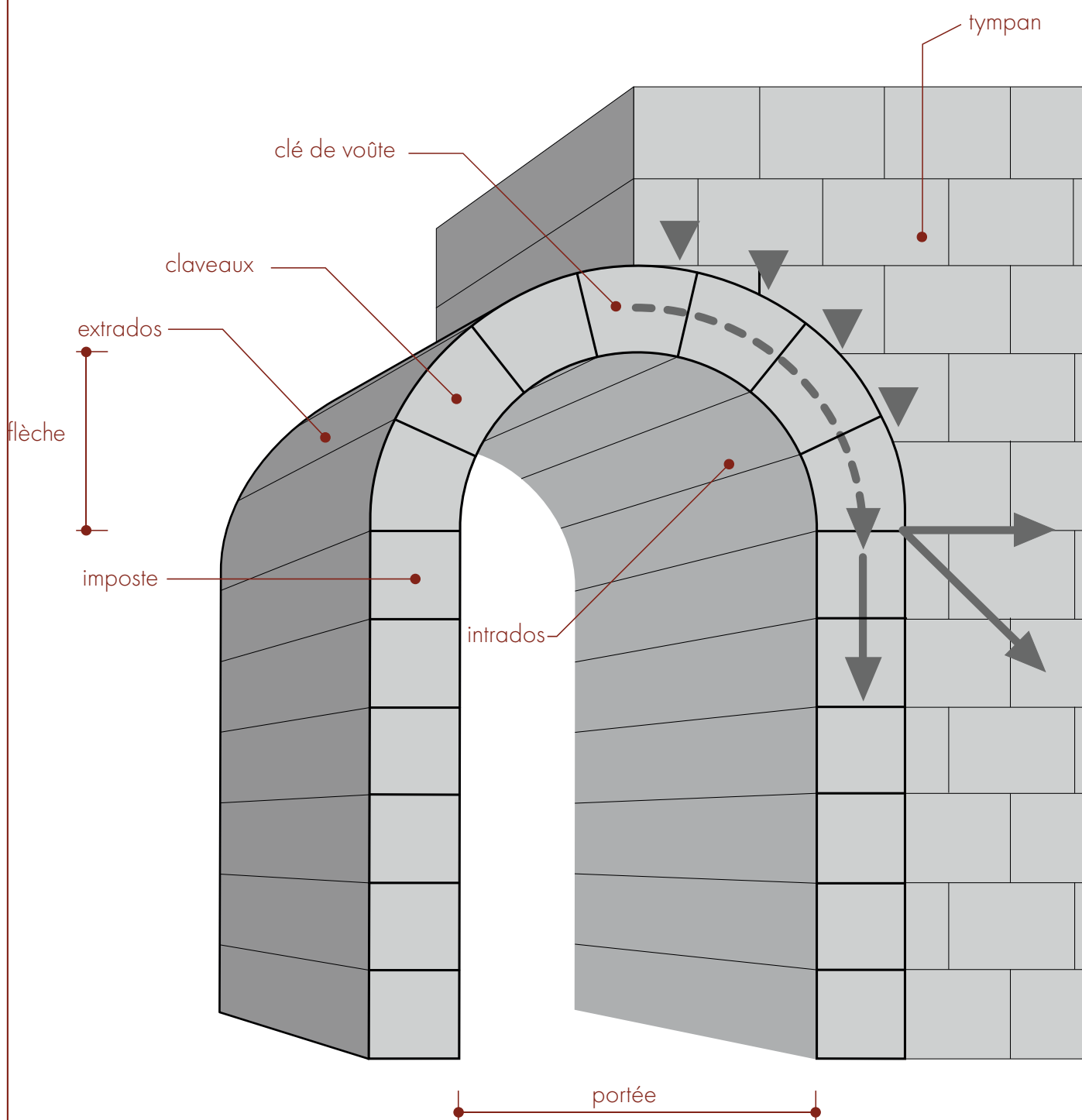
Schéma d'un arc et du montage de ses claveaux (© Lusitana, MesserWoland, Kilom691)
