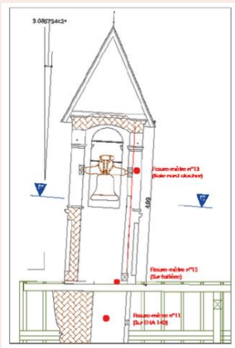
Coupe sur le déversement du clocher
