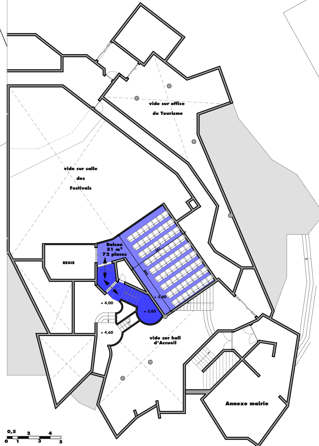
PLAN ETAGE
